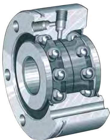
Rodamientos para husillos roscados.
