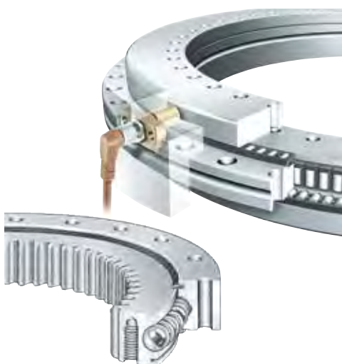
Rodamientos de precisión para cargas combinadas y coro- nas de precisión VSI
