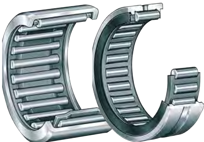
Casquillos de agujas con y sin fondo.
